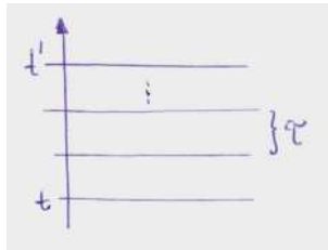
Abbildung 4.14: Teilintervalle.
