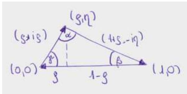
Abbildung 4.9: Das Unitaritätsdreieck.
