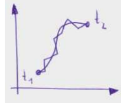
Abbildung 4.12: Trajektorie.
